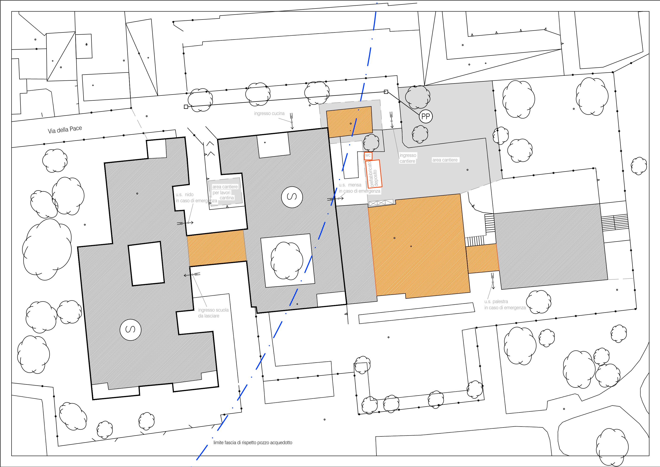
Layout del cantiere - dal 14.09.2026 (scala 1:200)
